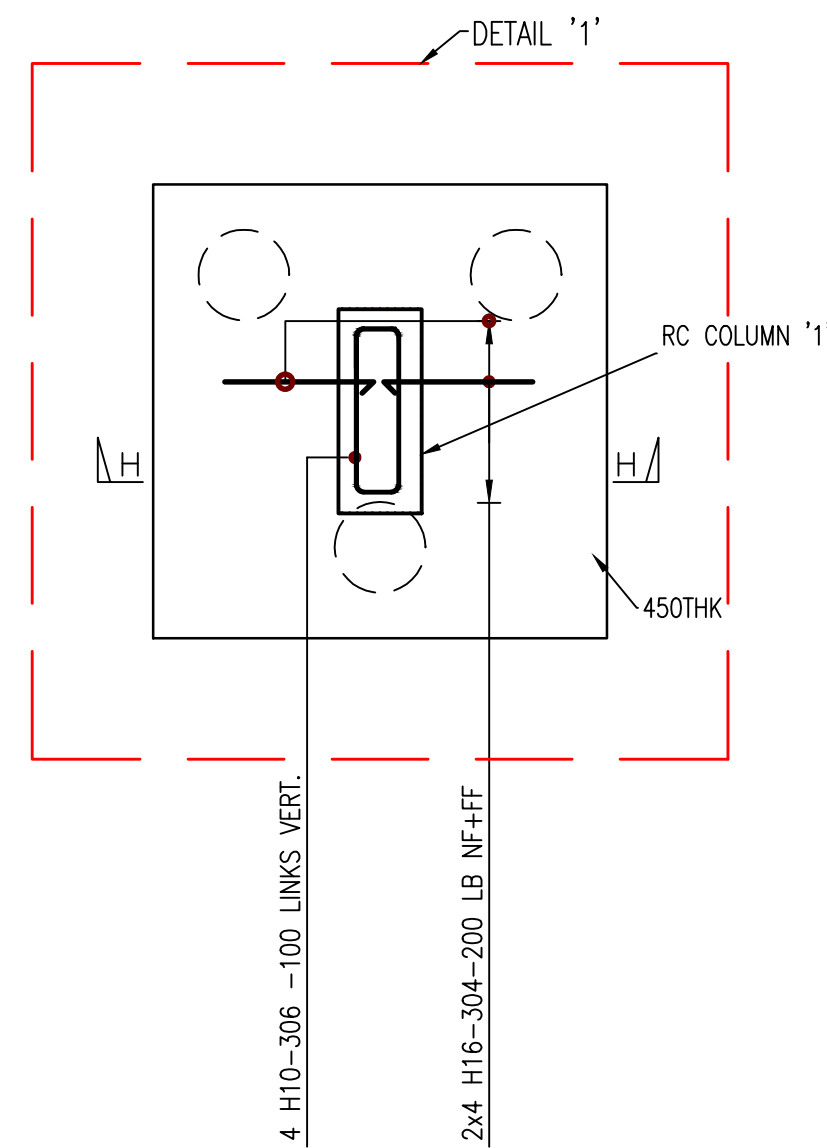
DETAIL '1' 7No. SCALE 1:25
